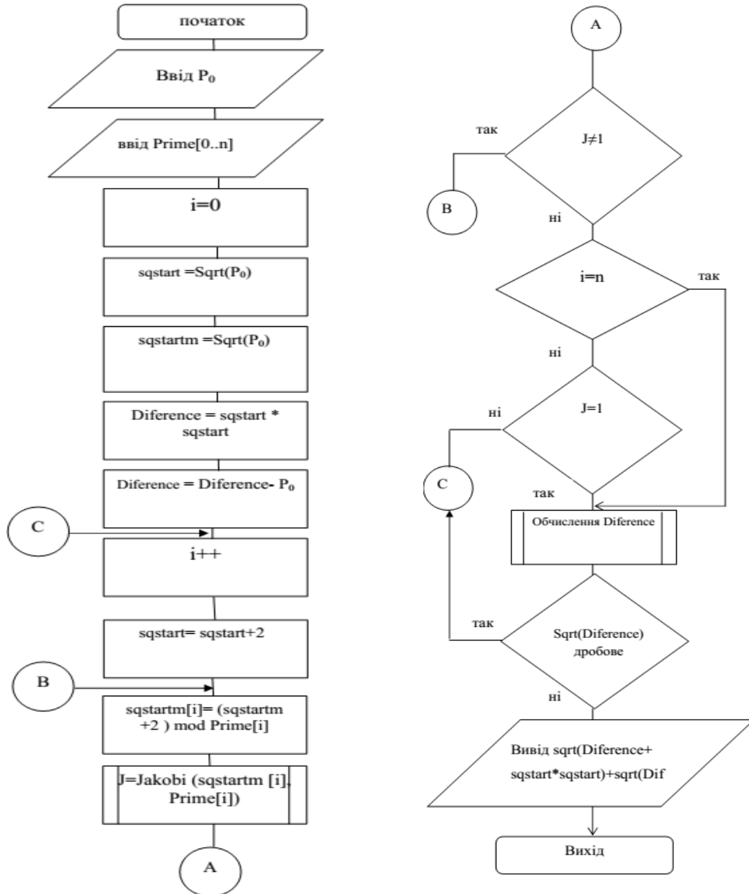
Рисунок 1 – Блок-схема модифікованого алгоритму факторизації
