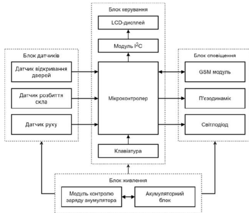
Рис. 1 – Структурна схема побутової охоронної системи
