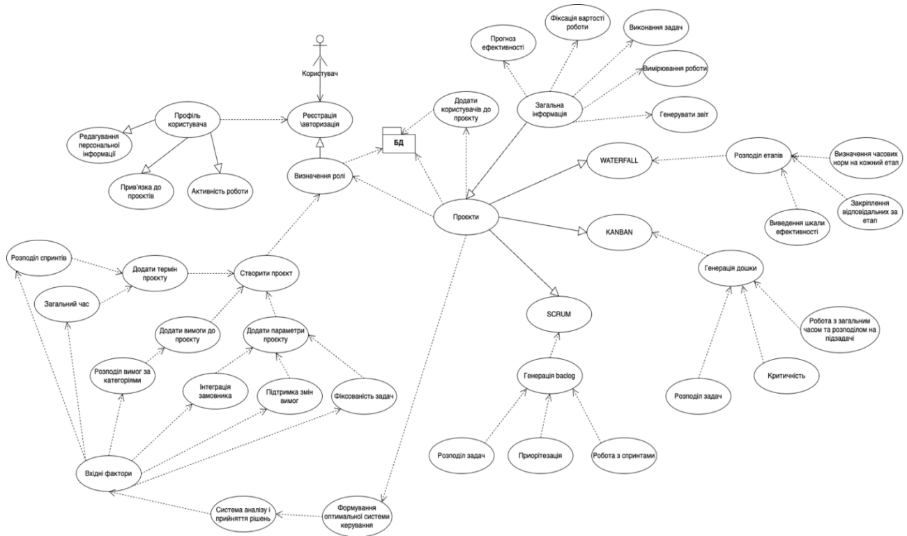
Рисунок 1 – Діаграма варіантів використання програмного засобу
