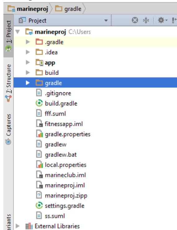
Рисунок 1 – Загальна файлова структура проекту у середовищі розробки Android Studio
