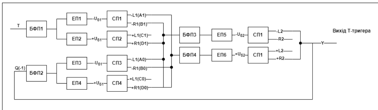
Рис. 1 – Схема трійкового Т-тригера
